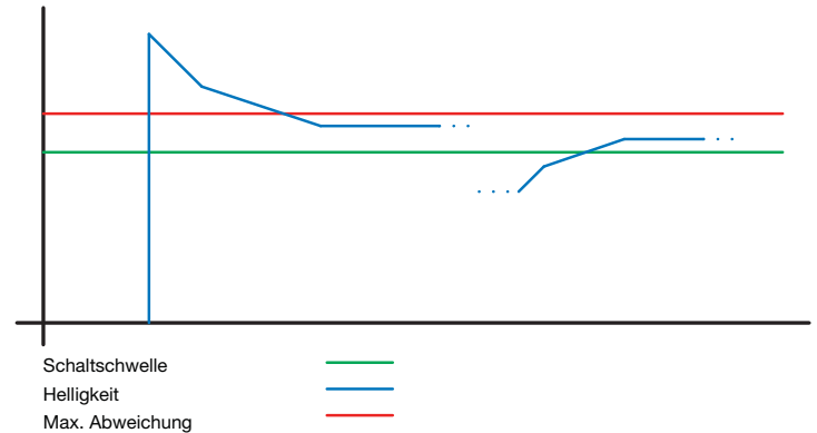
Abbildung 3: Bereich Konstantlichtregelung ausgegeregelt
